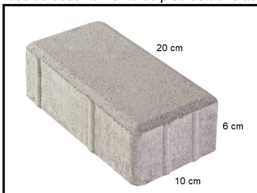
Figura 02 – Piso intertravado de concreto (Paver)
